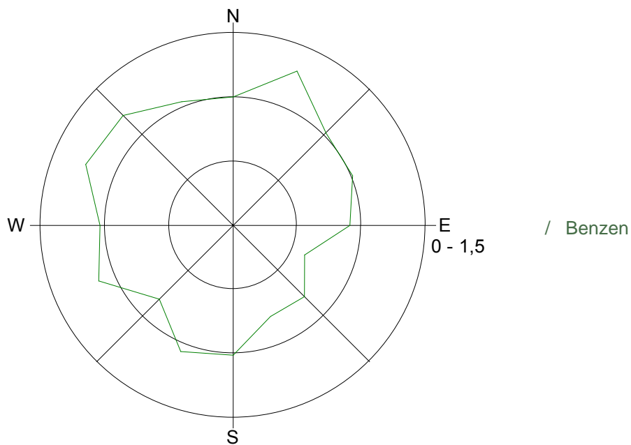
Slika 6: Roža onesnaženosti – benzen, oktober 2017.
