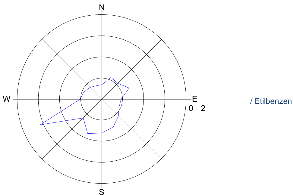
Slika 7: Roža onesnaženosti – etilbenzen, oktober 2017.
