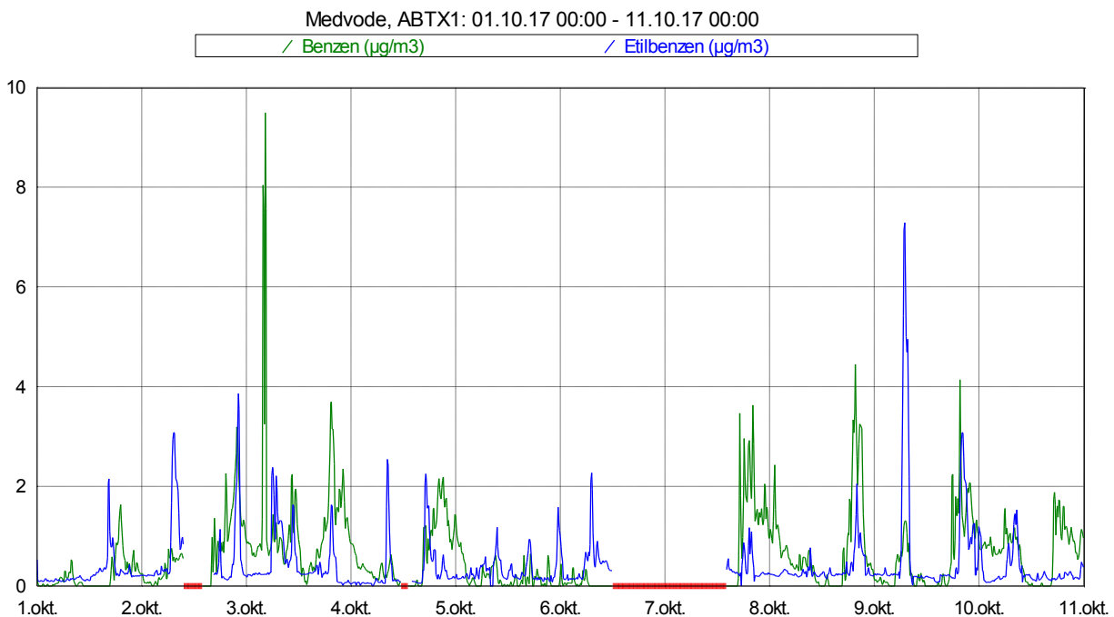
Slika 3: Imisijske koncentracije benzena in etilbenzena med vključno 1. 10. in 10. 10. 2017.
