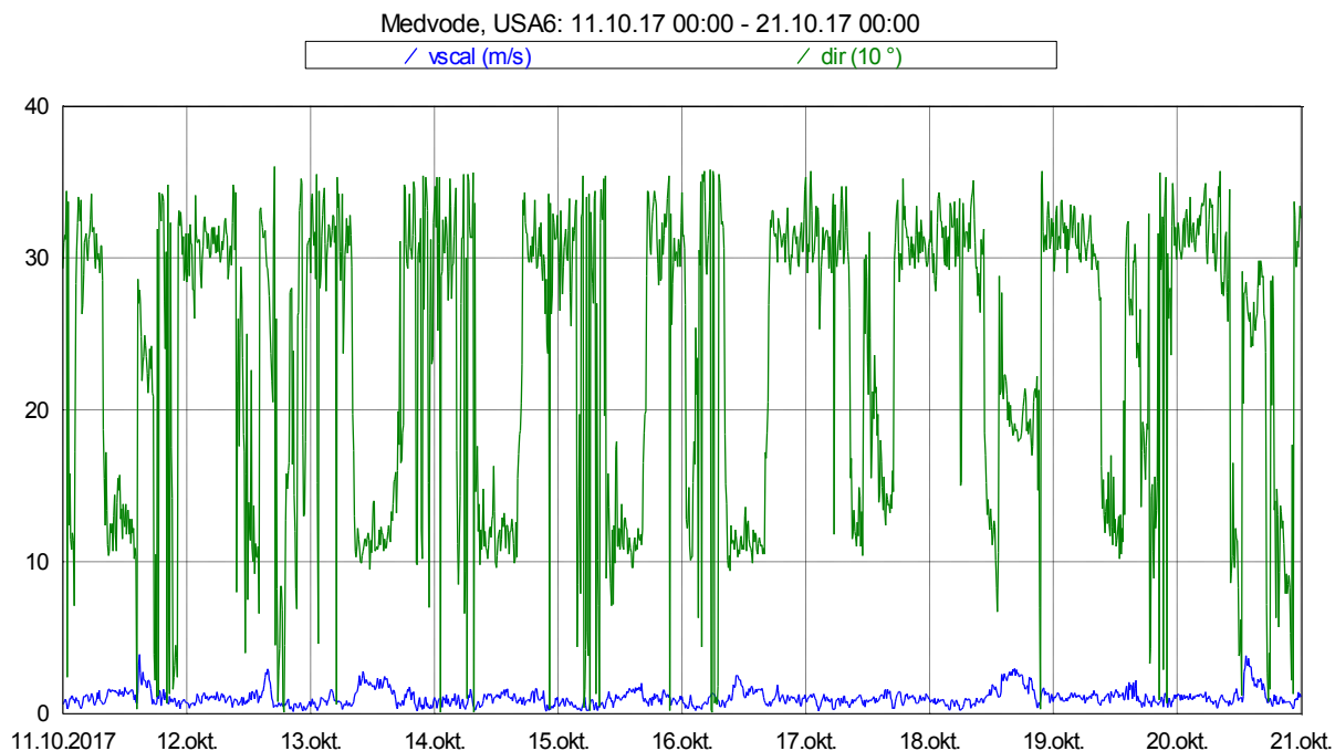
Slika 17: Smer in hitrost vetra med 11. 10. in 20. 10. 2017.
