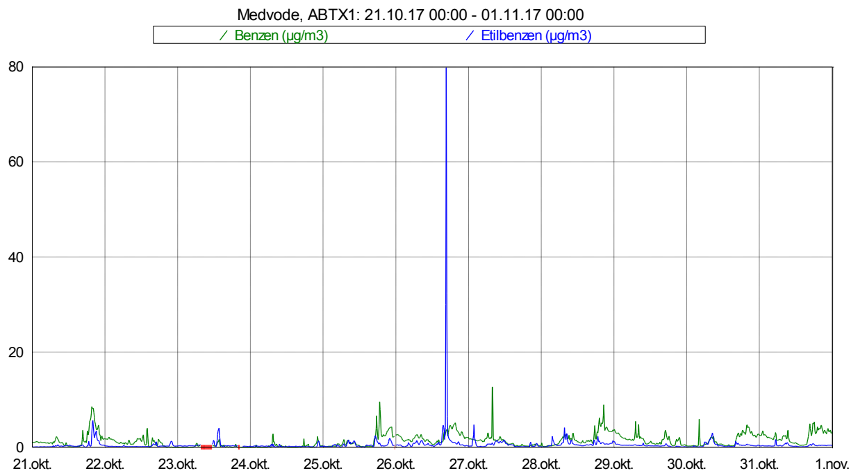
Slika 5: Imisijske koncentracije benzena in etilbenzena med vključno 21. 10. in 31. 10. 2017.
