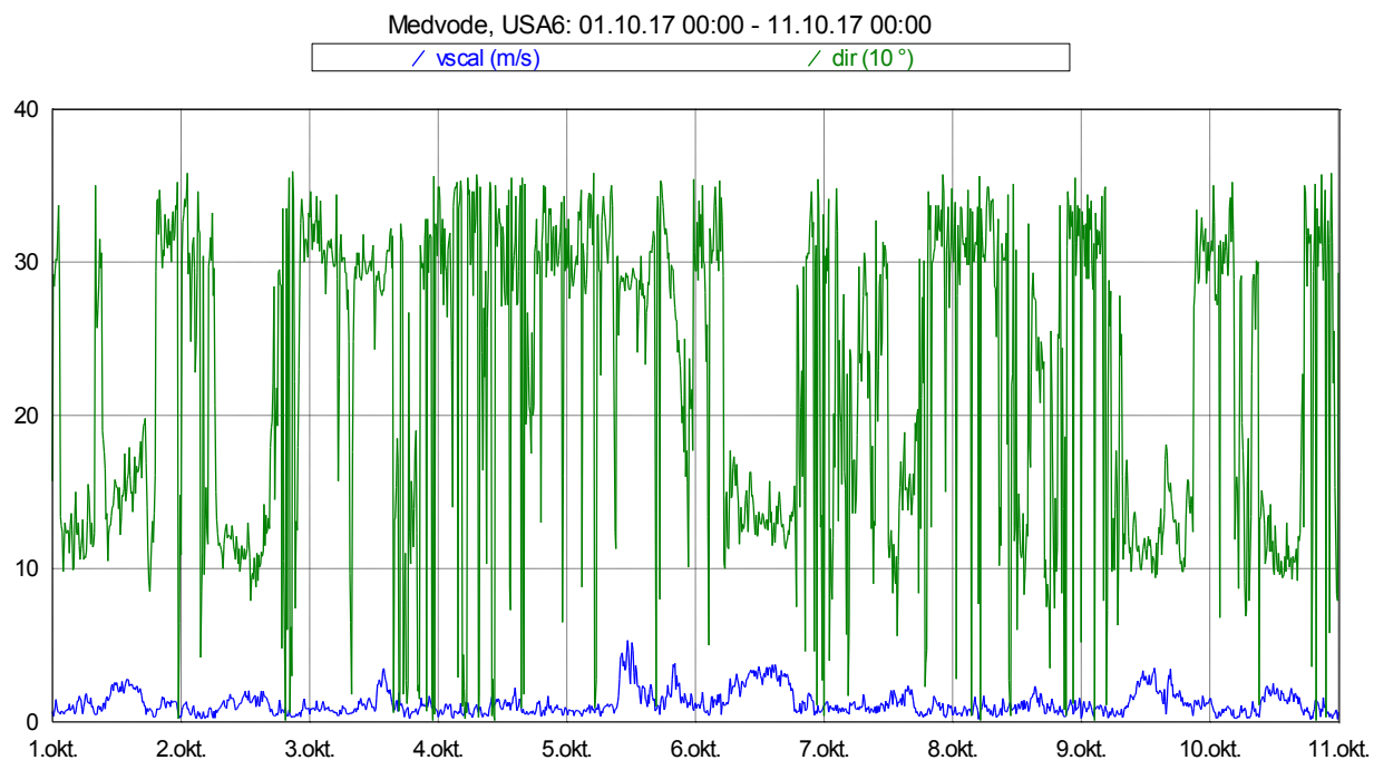
Slika 16: Smer in hitrost vetra med 1. 10. in 10. 10. 2017.
