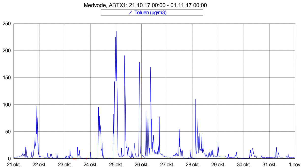
Slika 10: Imisijske koncentracije toluena med vključno 21. 9. in 30. 9. 2017.
