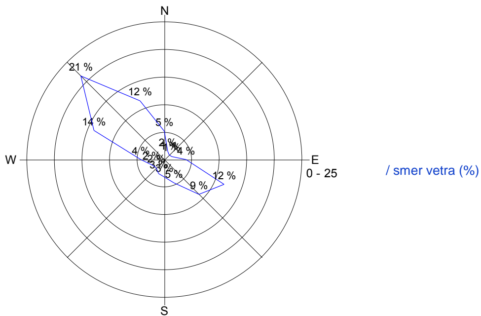
Slika 19: Roža vetrov, oktober 2017.
