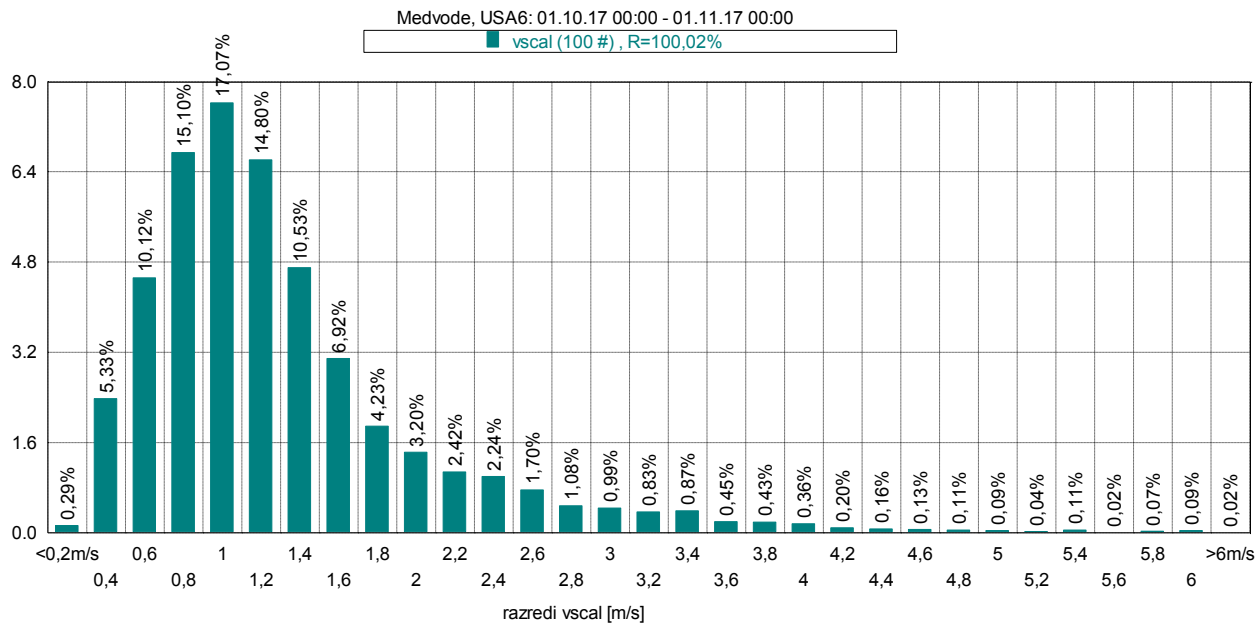
Slika 20: Frekvenčna porazdelitev po hitrosti vetra, oktober 2017.
