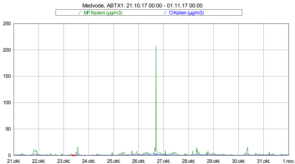
Slika 14: Imisijske koncentracije ksilenov med vključno 21. 10. in 31. 10. 2017.
