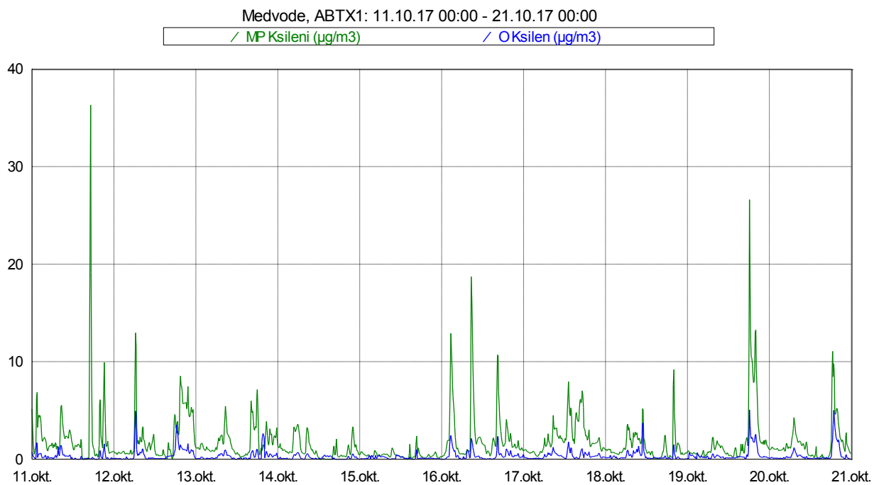
Slika 13: Imisijske koncentracije ksilenov med vključno 11. 10. in 20. 10. 2017.
