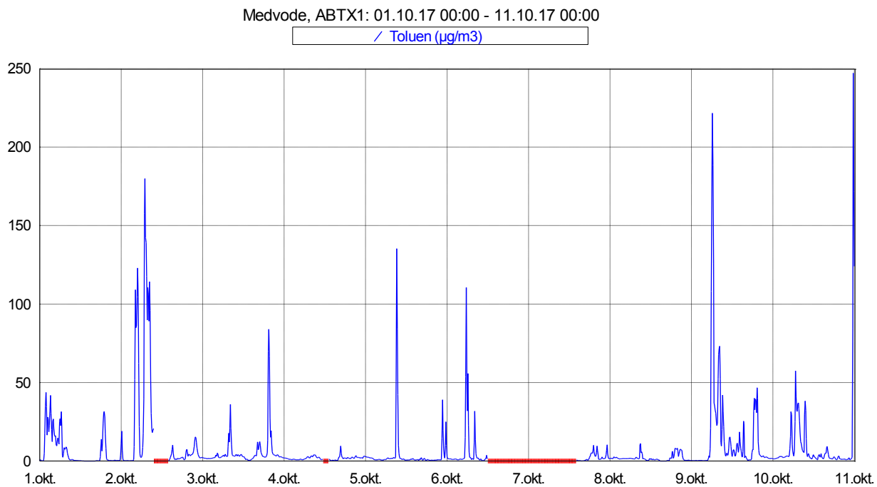
Slika 8: Imisijske koncentracije toluena med vključno 1. 10. in 10. 10. 2017.
