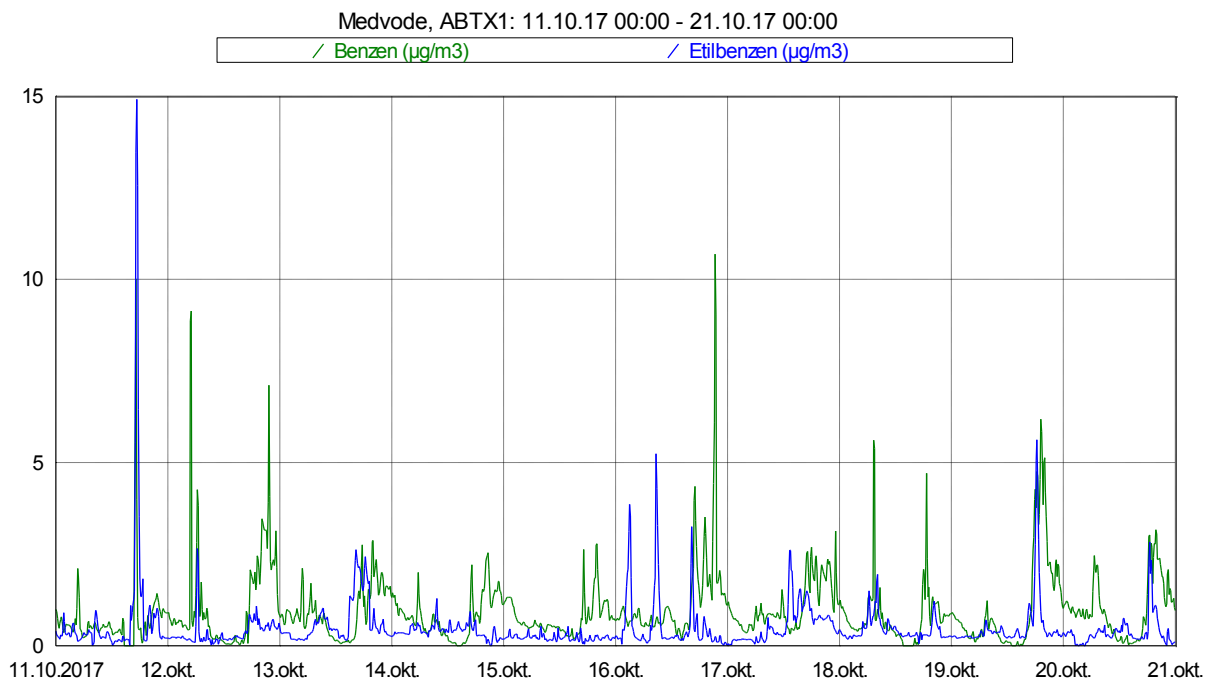
Slika 4: Imisijske koncentracije benzena in etilbenzena med vključno 11. 10. in 20. 10. 2017.
