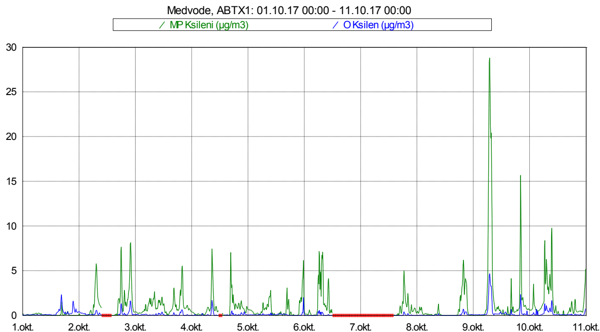
Slika 12: Imisijske koncentracije ksilenov med vključno 1. 10. in 10. 10. 2017.
