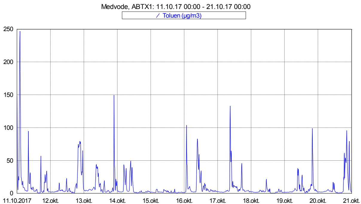
Slika 9: Imisijske koncentracije toluena med vključno 11. 10. in 20. 10. 2017.
