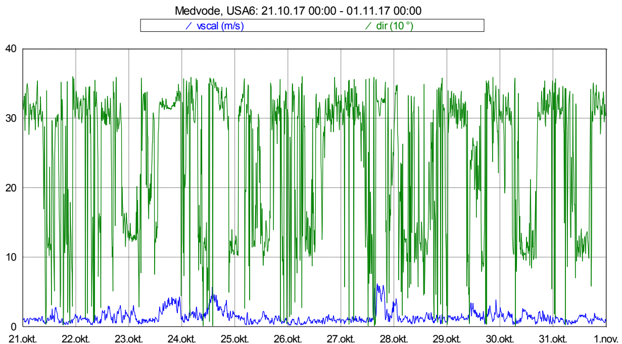
Slika 18: Smer in hitrost vetra med 21. 10. in 31. 10. 2017.
