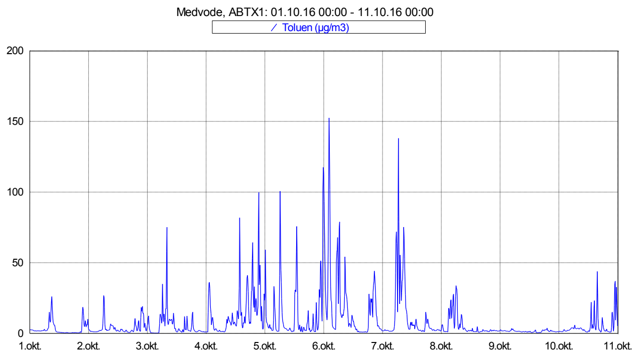
Slika 8: Imisijske koncentracije toluena med vključno 1. 10. 2016 in 10. 10. 2016.
