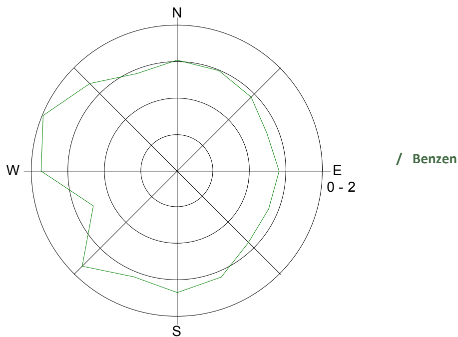
Slika 6: Roža onesnaženosti – benzen, oktober 2016.
