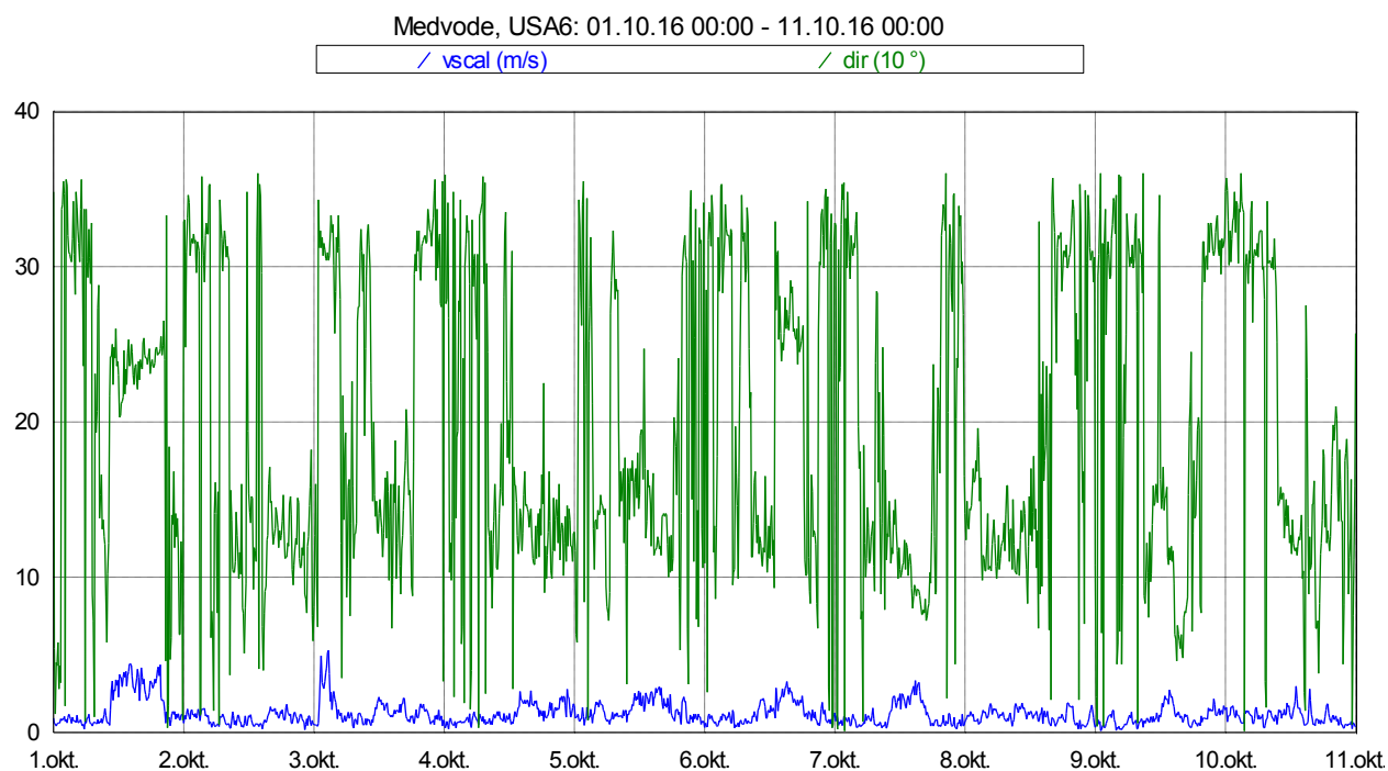
Slika 16: Smer in hitrost vetra med 1. 10. 2016 in 10. 10. 2016.
