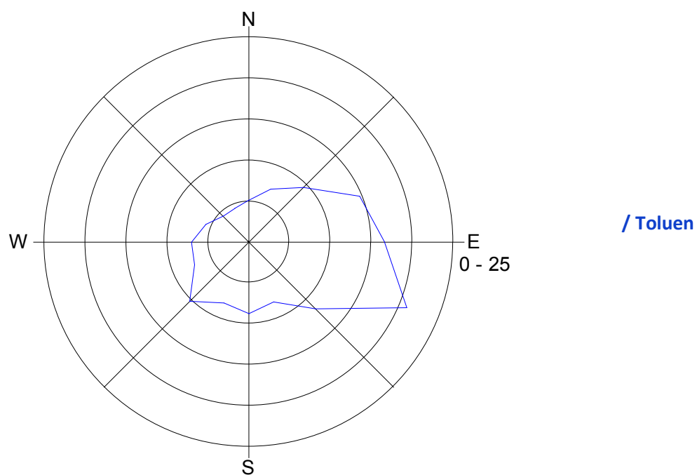
Slika 11: Roža onesnaženost - toluen, oktober 2016.
