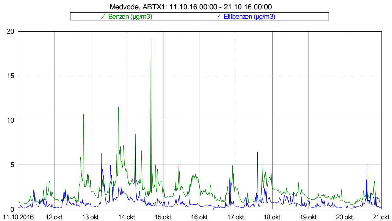
Slika 4: Imisijske koncentracije benzena in etilbenzena med 11. 10. 2016 in 20. 10. 2016.
