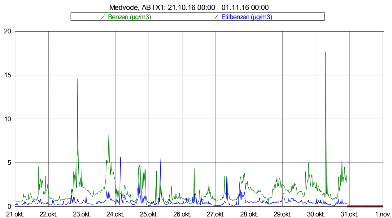
Slika 5: Imisijske koncentracije benzena in etilbenzena med 21. 10. 2016 in 31. 10. 2016.
