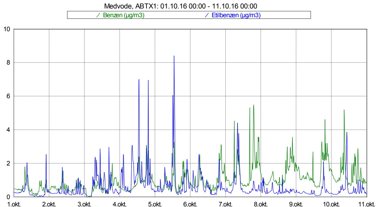
Slika 3: Imisijske koncentracije benzena in etilbenzena med vključno 1. 10. 2016 in 10. 10. 2016.
