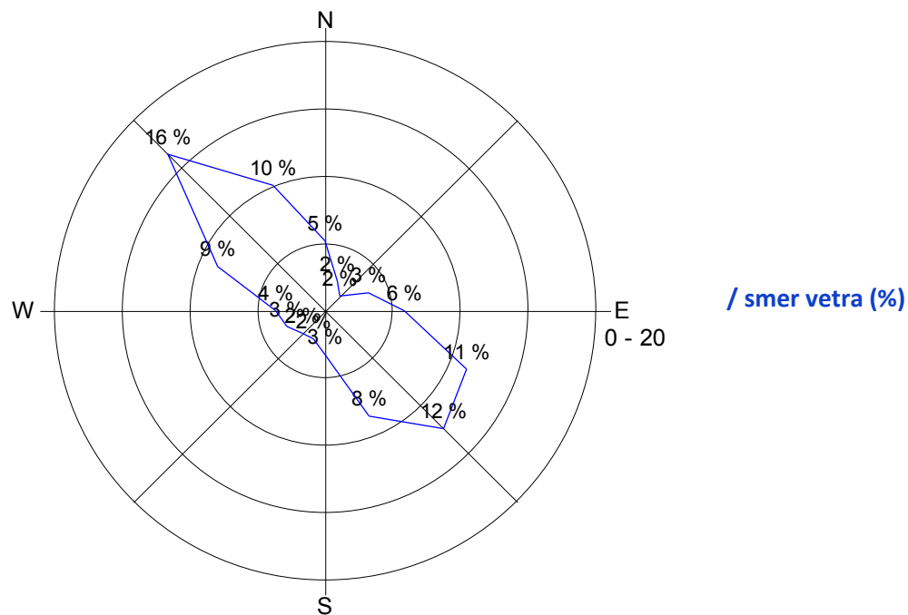
Slika 18: Smer in hitrost vetra med 21. 10. 2016 in 31. 10. 2016.
