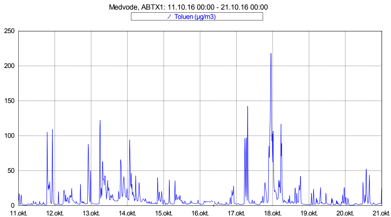
Slika 9: Imisijske koncentracije toluena med 11. 10. 2016 in 20. 10. 2016.
