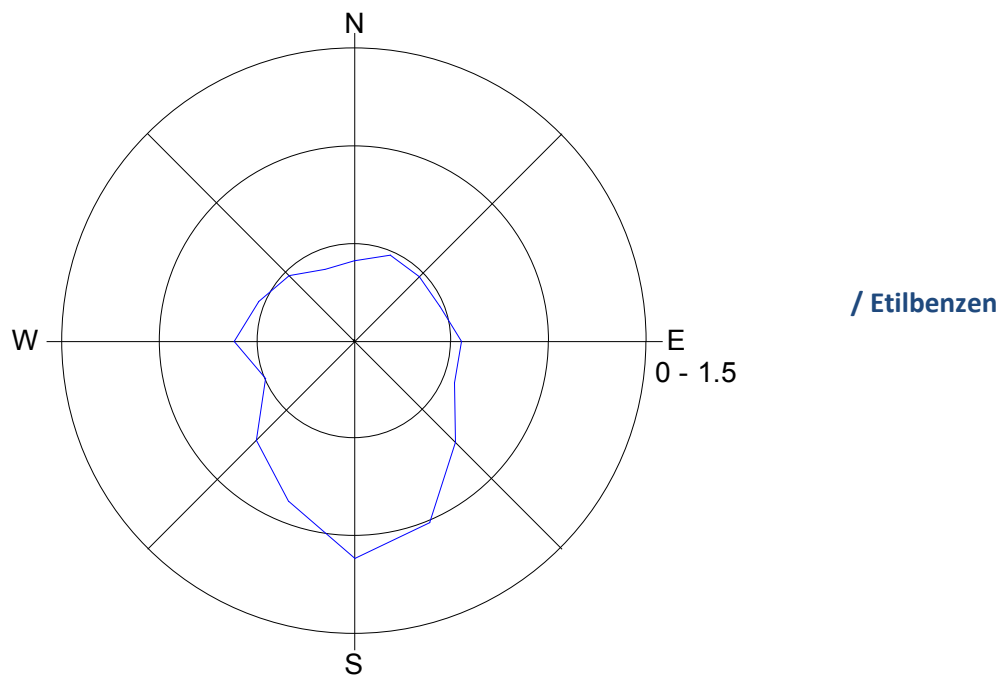
Slika 7: Roža onesnaženosti – etilbenzen, oktober 2016.
