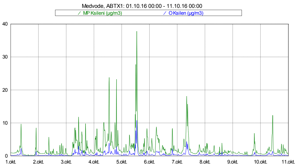
Slika 12: Imisijske koncentracije M&P in O ksilena med vključno 1. 10. 2016 in 10. 10. 2016.
