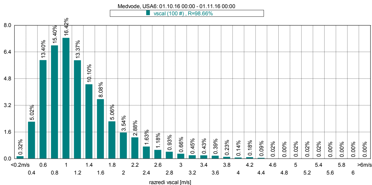
Slika 20: Frekvenčna porazdelitev po hitrosti vetra, oktober 2016.
