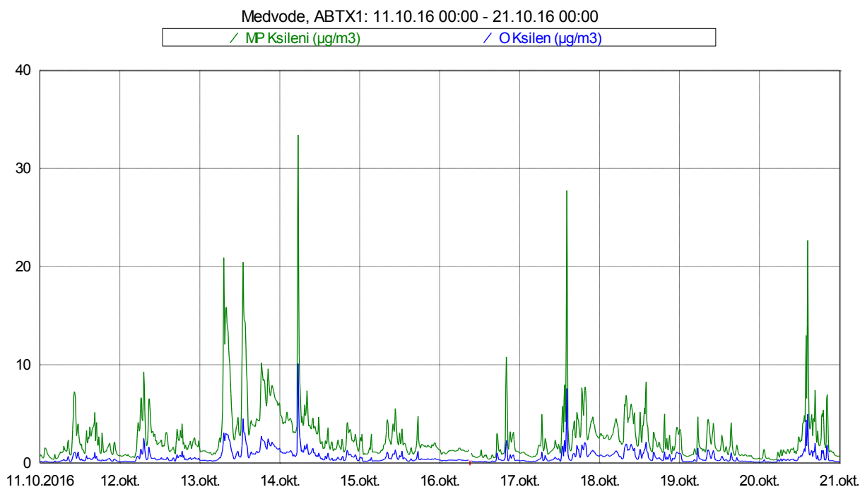
Slika 13: Imisijske koncentracije M&P in O ksilena med 11. 10. 2016 in 20. 10. 2016.
