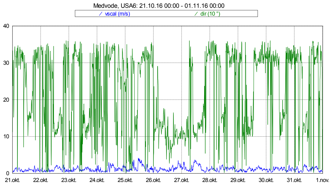
Slika 18: Smer in hitrost vetra med 21. 10. 2016 in 31. 10. 2016.
