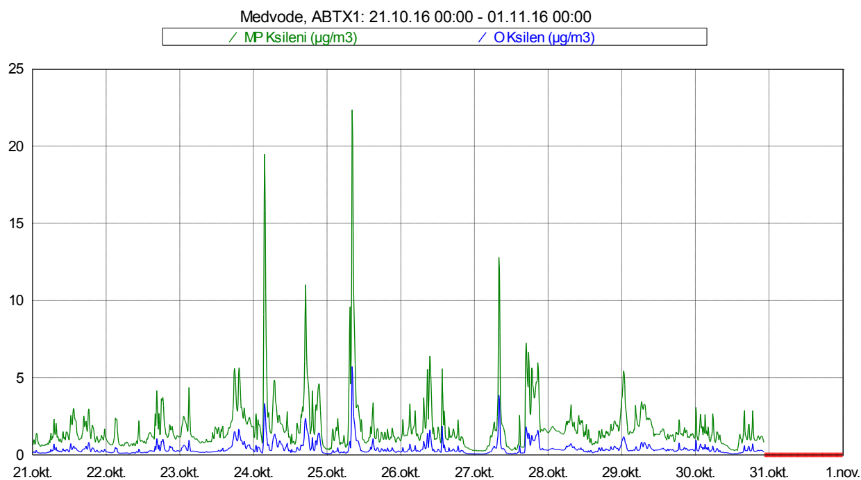
Slika 14: Imisijske koncentracije M&P in O ksilena med 21. 10. 2016 in 31. 10. 2016.
