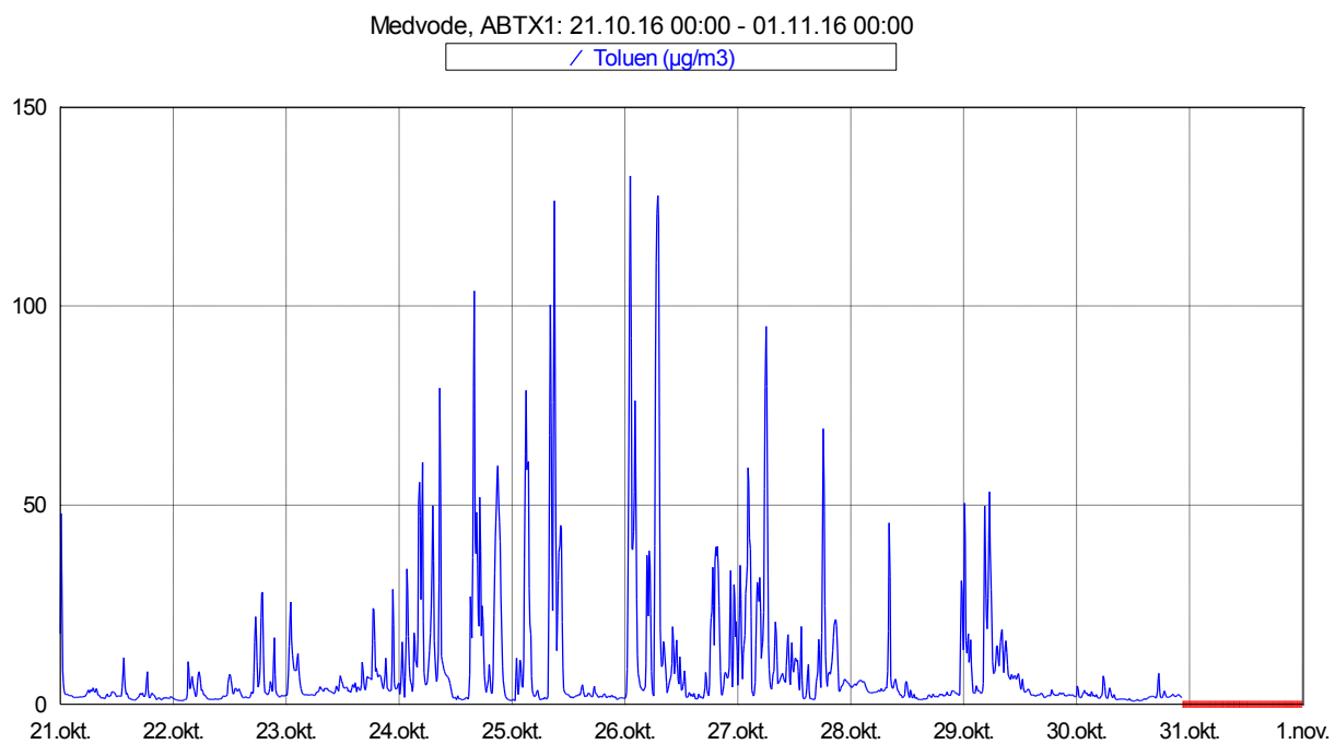
Slika 10: Imisijske koncentracije toluena med 21. 10. 2016 in 31. 10. 2016.
