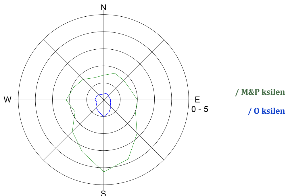
Slika 15: Roža onesnaženosti - M & P ksilen in O ksilen, oktober 2016.
