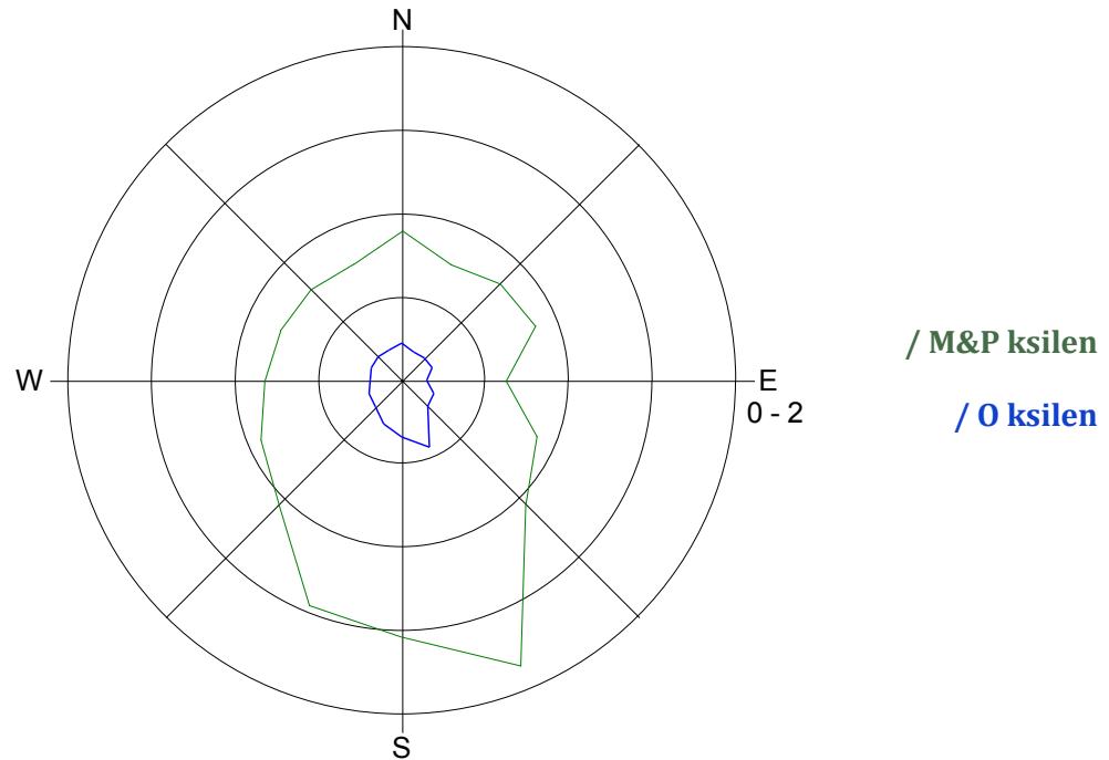
Slika 15: Roža onesnaženosti - M & P ksilen in O ksilen, julij 2015.
