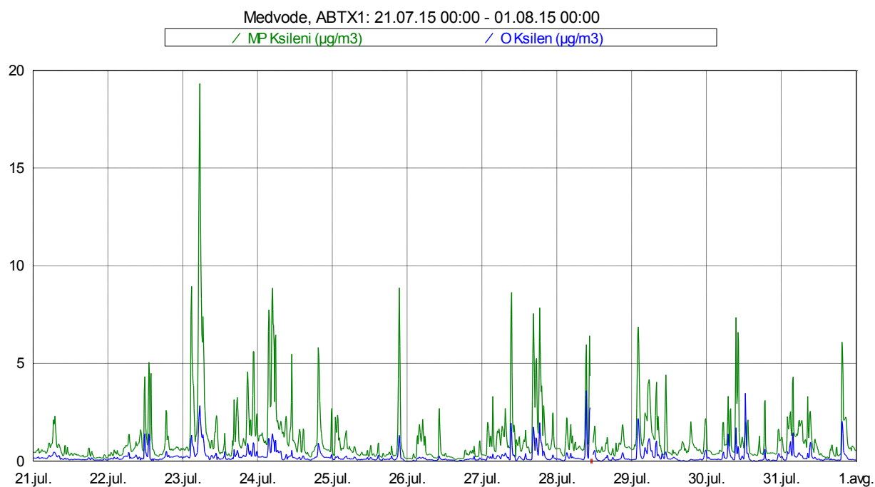
Slika 14: Imisijske koncentracije M&P in O ksilena med 21. 7. 2015 in 31. 7. 2015.
