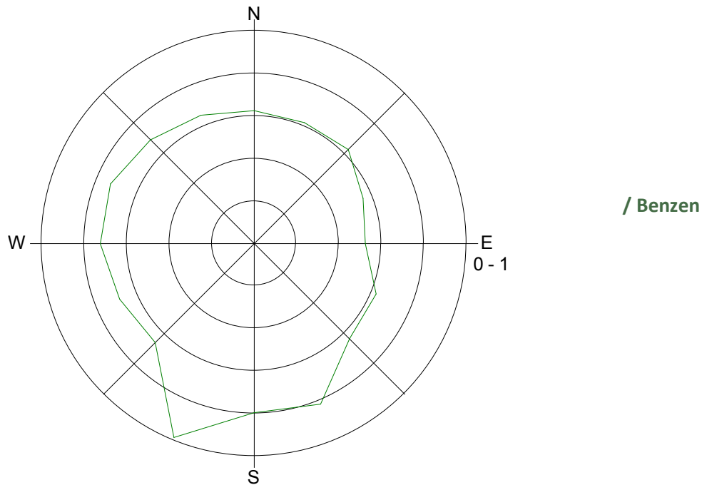
Slika 6: Roža onesnaženosti – benzen, julij 2015.
