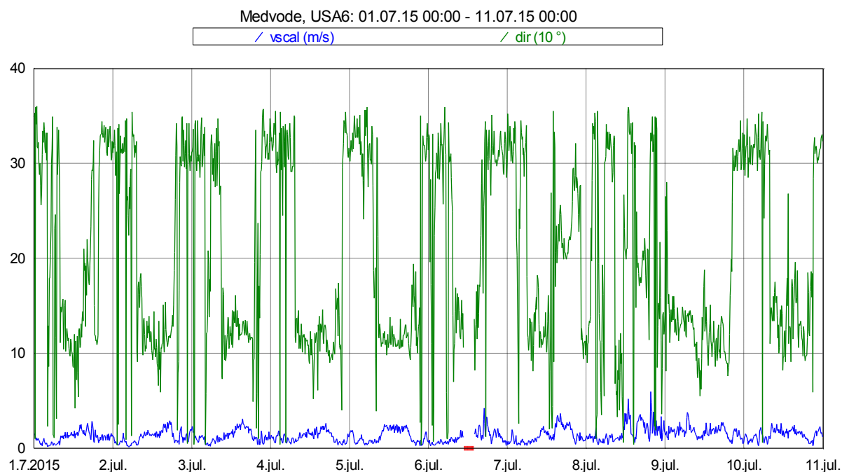
Slika 16: Smer in hitrost vetra med 1. 7. 2015 in 10. 7. 2015.
