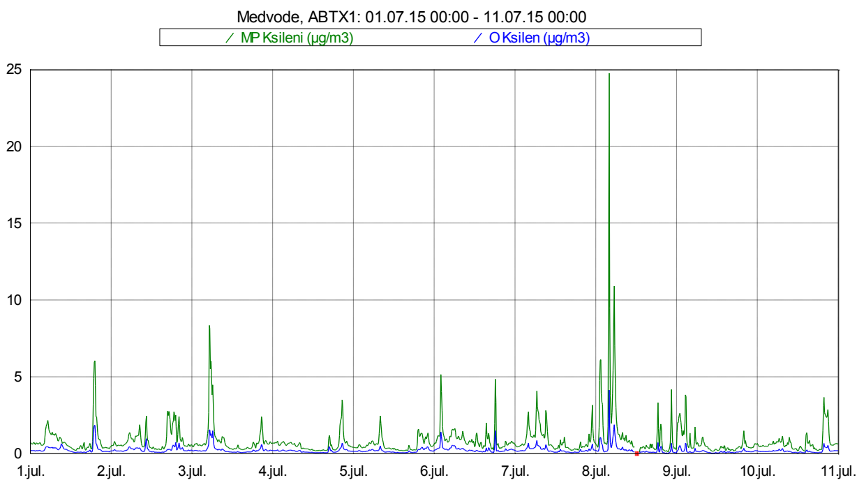
Slika 12: Imisijske koncentracije M&P in O ksilena med vključno 1. 7. 2015 in 10. 7. 2015.
