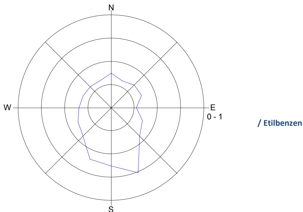
Slika 7: Roža onesnaženosti – etilbenzen, julij 2015.
