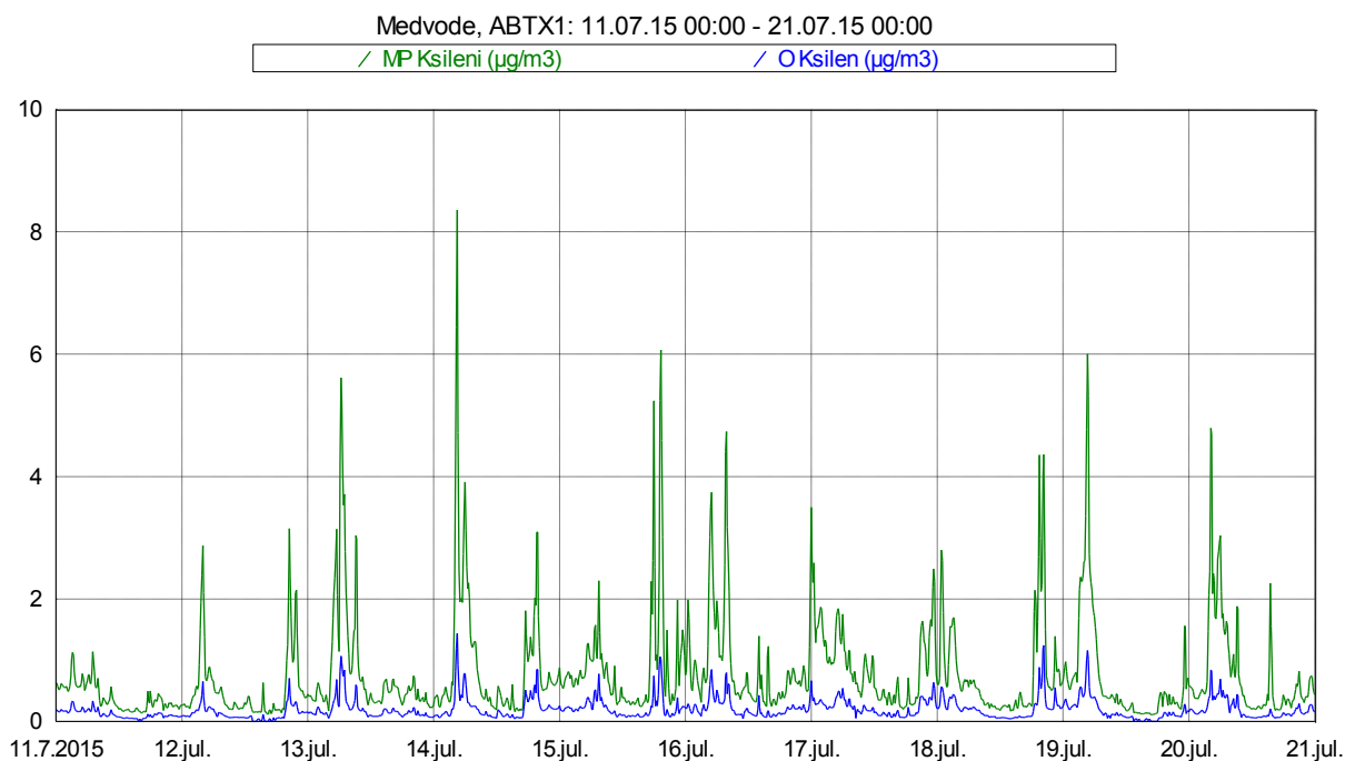
Slika 13: Imisijske koncentracije M&P in O ksilena med 11. 7. 2015 in 20. 7. 2015.
