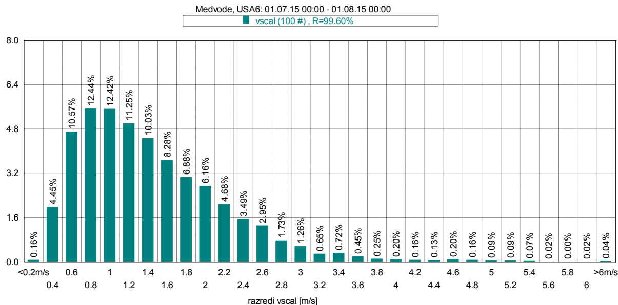
Slika 20: Frekvenčna porazdelitev po hitrosti vetra, julij 2015.
