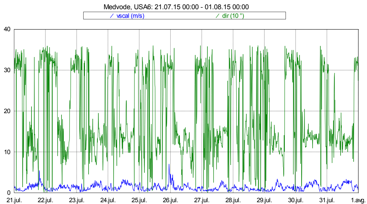
Slika 18: Smer in hitrost vetra med 21. 7. 2015 in 31. 7. 2015.
