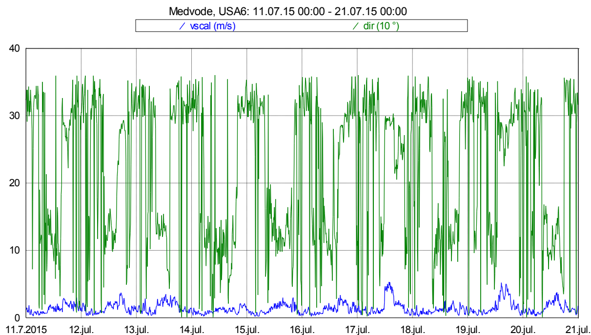
Slika 17: Smer in hitrost vetra med 11. 7. 2015 in 20. 7. 2015.
