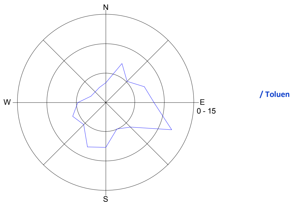
Slika 11: Roža onesnaženost - toluen, julij 2015.
