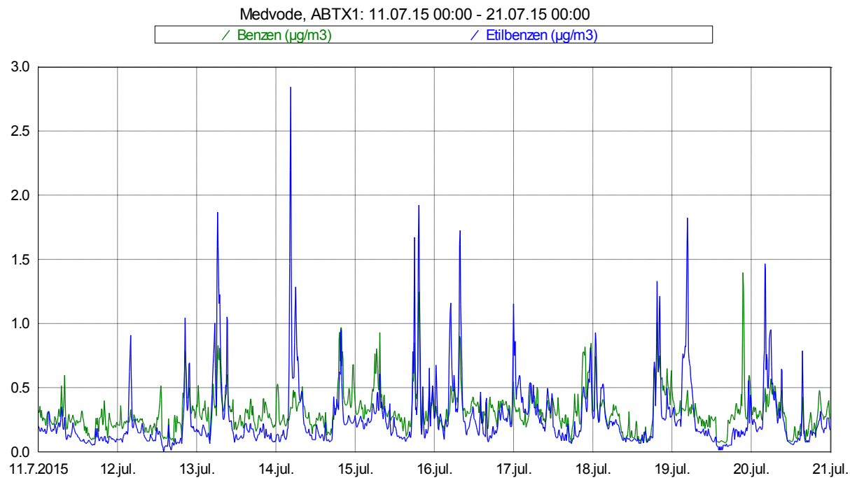
Slika 4: Imisijske koncentracije benzena in etilbenzena med 11. 7. 2015 in 20. 7. 2015.
