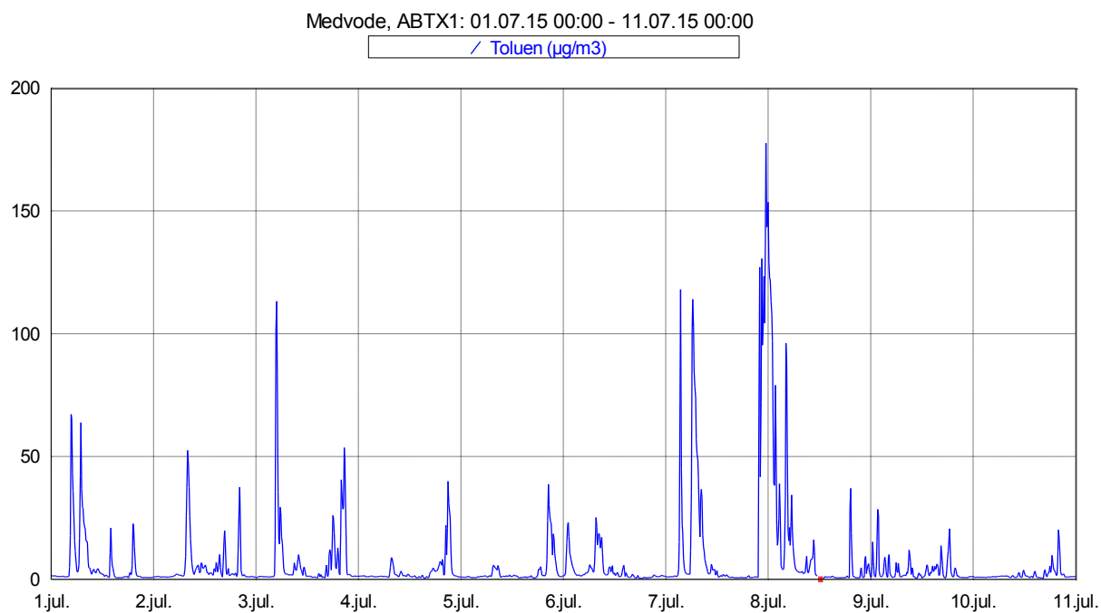
Slika 8: Imisijske koncentracije toluena med vključno 1. 7. 2015 in 10. 7. 2015.
