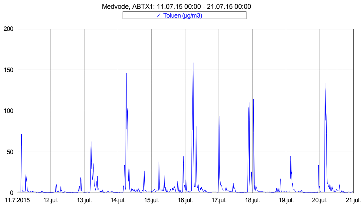
Slika 9: Imisijske koncentracije toluena med 11. 7. 2015 in 20. 7. 2015.
