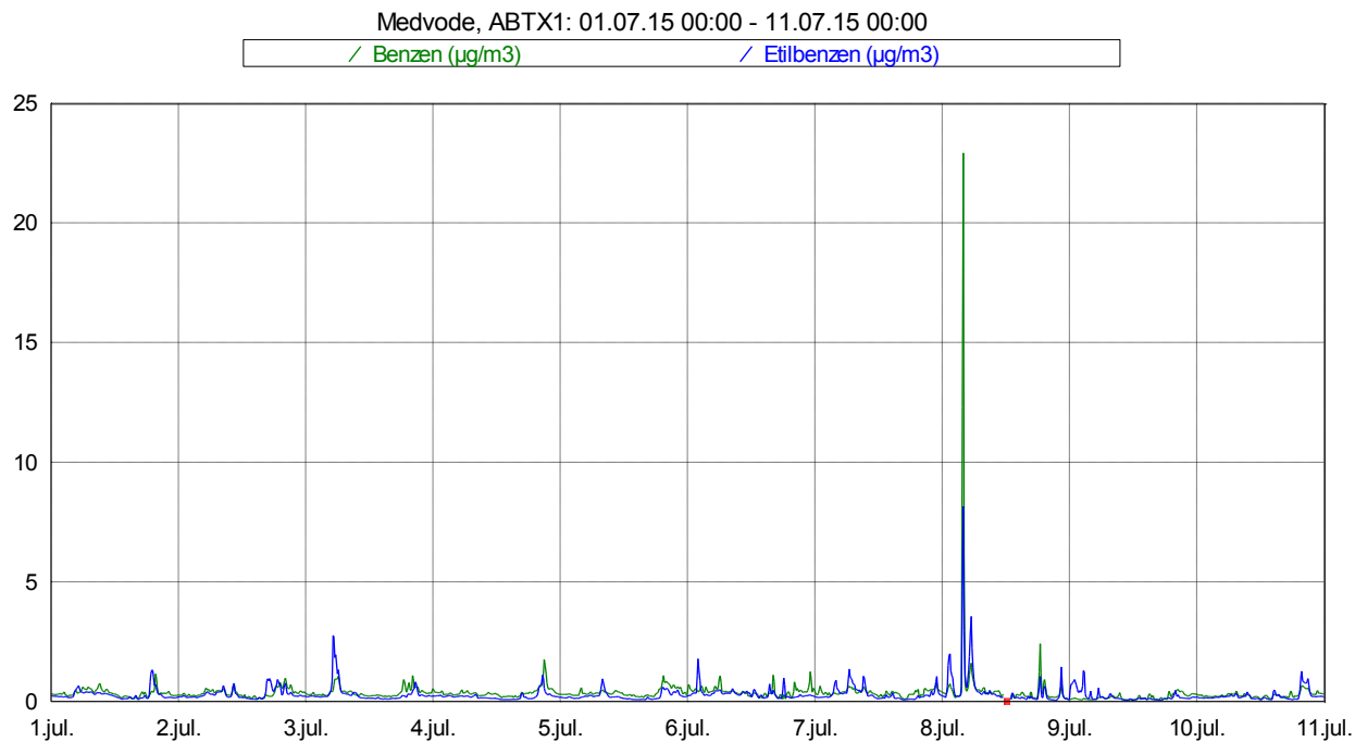
Slika 3: Imisijske koncentracije benzena in etilbenzena med vključno 1. 7. 2015 in 10. 7. 2015.
