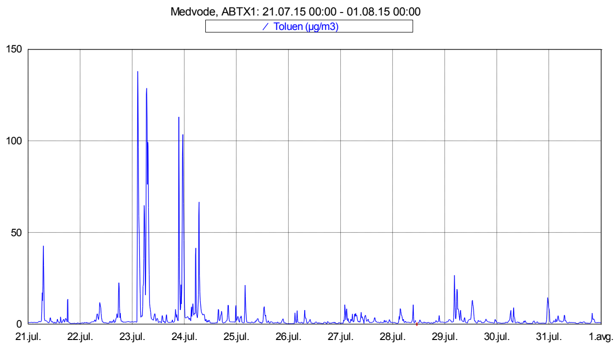
Slika 10: Imisijske koncentracije toluena med 21. 7. 2015 in 31. 7. 2015.
