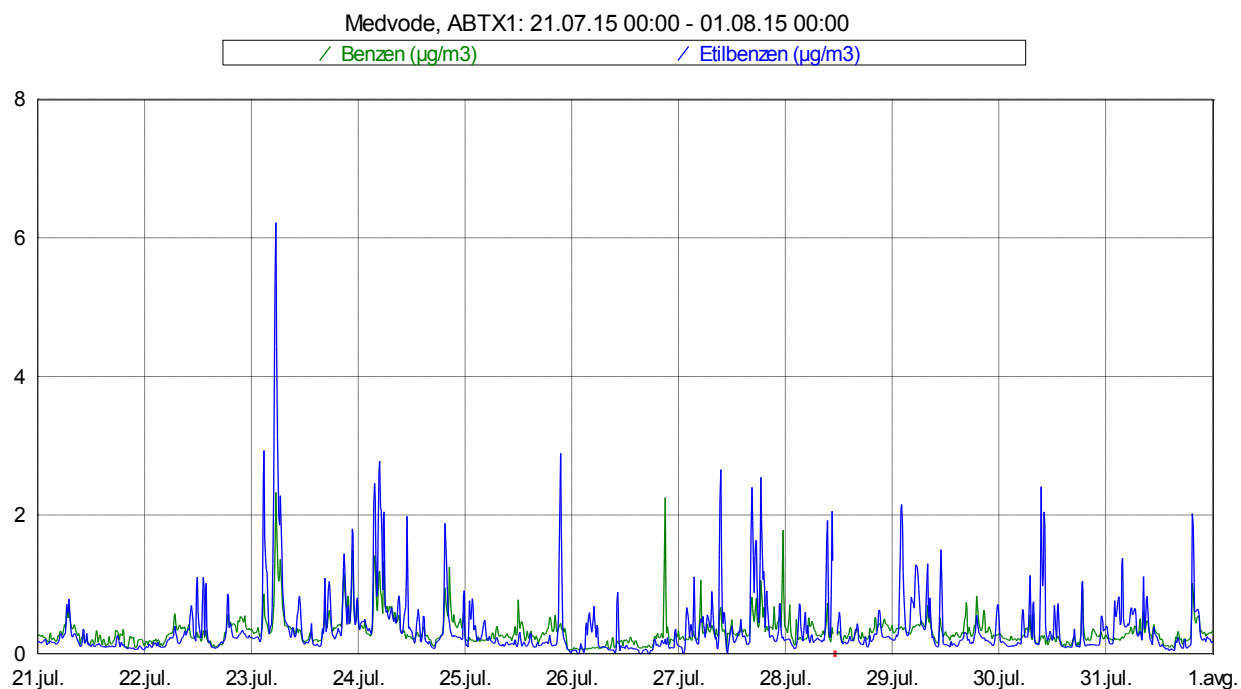
Slika 5: Imisijske koncentracije benzena in etilbenzena med 21. 7. 2015 in 31. 7. 2015.
