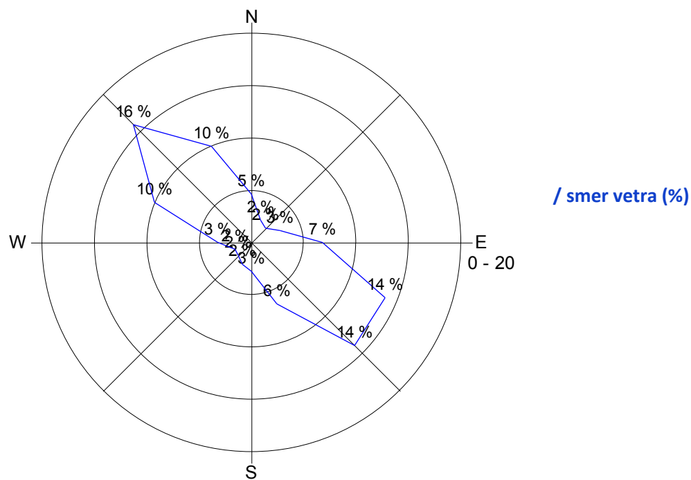
Slika 19: Roža vetrov, julij 2015.
